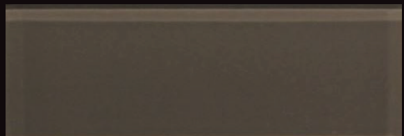
Vapor
